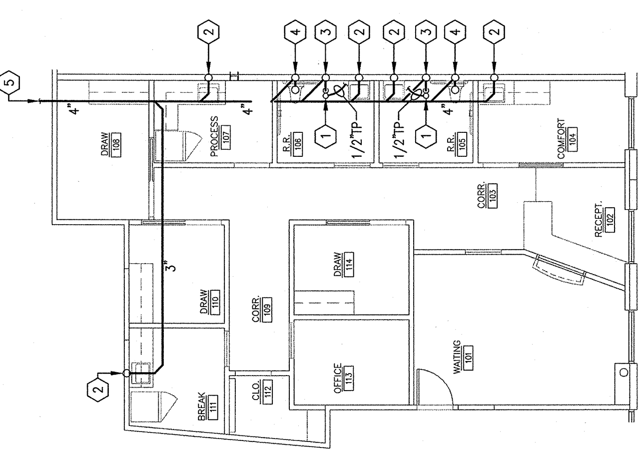
01 UNDERFLOOR PLAN - PLUMBING SCALE: 1/8" = 1'-0"
